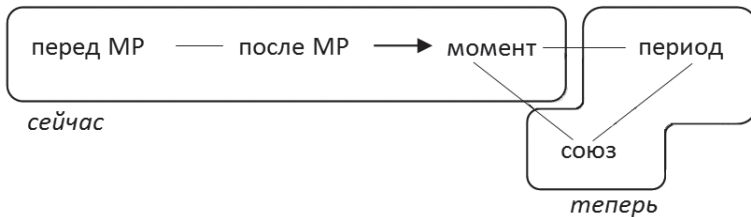
Схема 2. Семантическая карта теперь и сейчас начиная с 1880-х гг.
