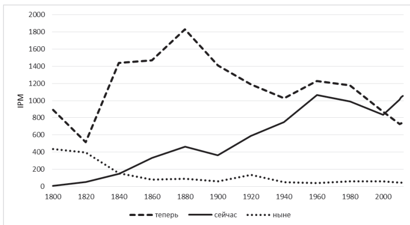
График 1. Количество словоупотреблений на миллион словоформ у теперь , сейчас и ныне . Данные НКРЯ, 1800–2012 гг.
