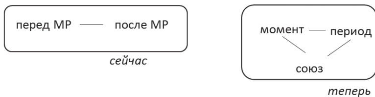
Схема 1. Семантические функции теперь и сейчас на начало XIX в.
