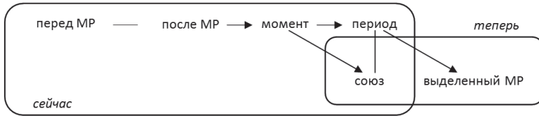
Схема 3. Предполагаемая ситуация, к которой ведут действующие тенденции
